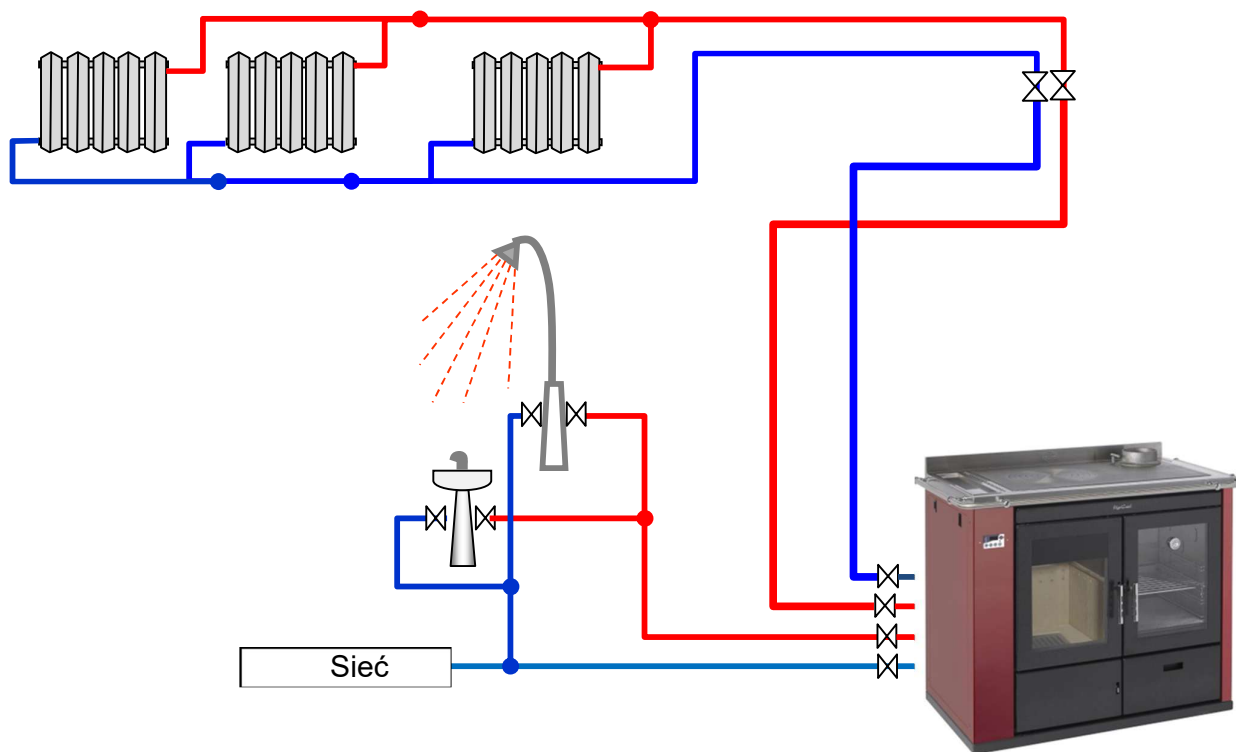
Typowa instalacja ogrzewania i ciepłej wody użytkowej z zainstalowaną termokuchnią.
