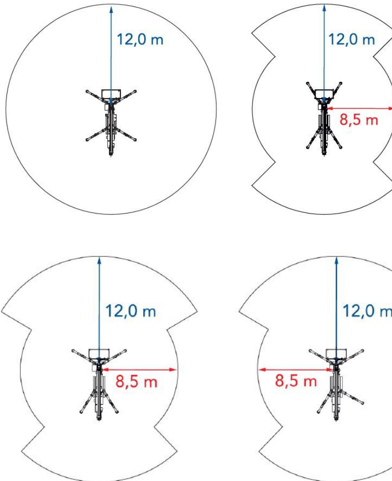
Diagramy zasięgu pracy dla poszczególnej konfiguracji rozłożenia podpór.
