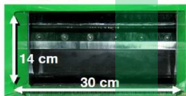
Wymiary otworu wejścia materiału
