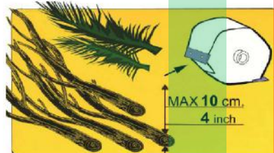
Wymiary otworu wejścia materiału
